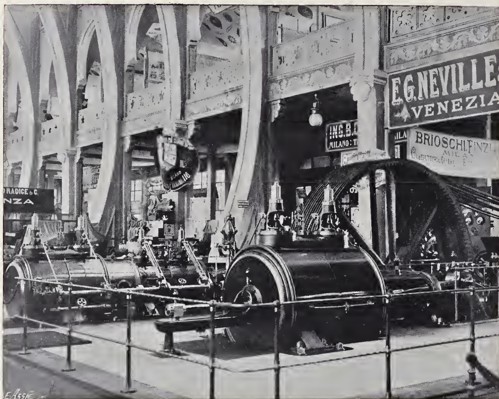
GALLERIA DEL LAVORO LE MOTRICI DELLA CASA E. G. NEVILLE E C. DI VENEZIA (Fot. Fratelli LOVAZZANO).
